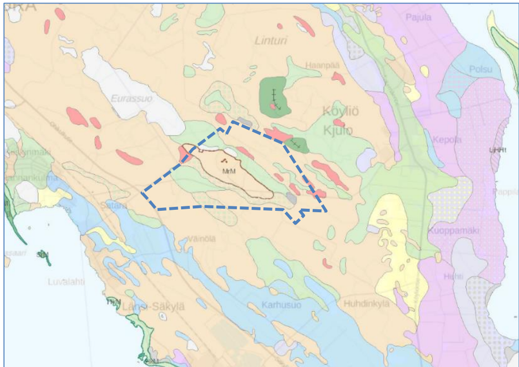
Kuva 2: Maaperäkartta (GTK). Suunnittelualan sijainti merkitty sinisellä katkoviivalla.
